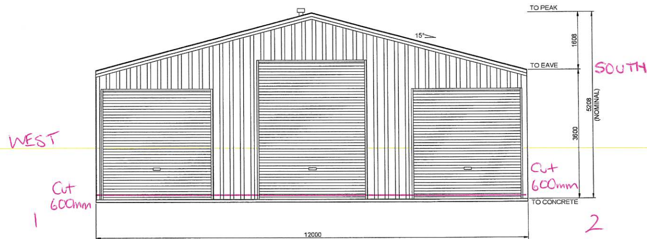
4 ENDWALL EXTERIOR ELEVATION SCALE: 1 = 100
